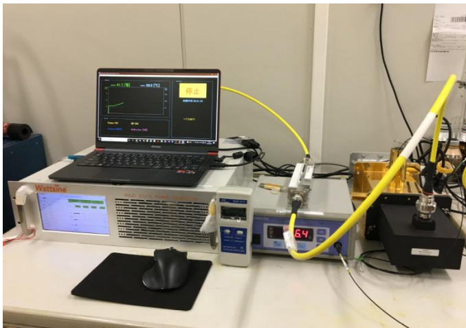
2.45GHz 200Wシングルモード加熱装置 温度制御機能付き
