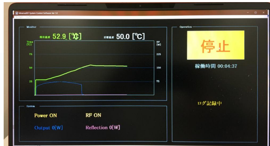
2.45GHz 300Wシングルモード加熱装置 温度制御機能付き
