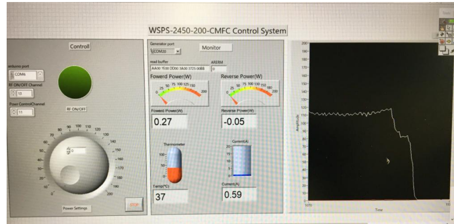
2.45GHz 200Wシングルモード加熱装置 温度制御機能付き
