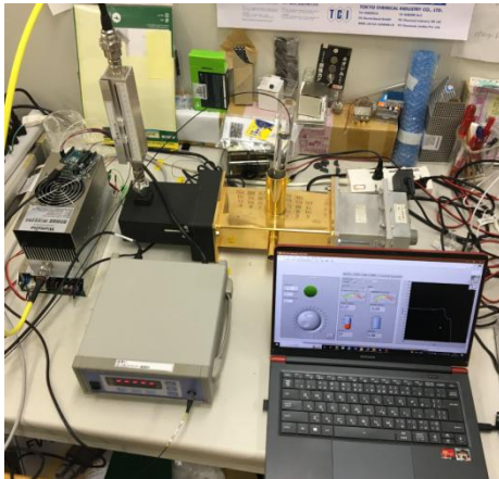
2.45GHz 200Wシングルモード加熱装置 温度制御機能付き
