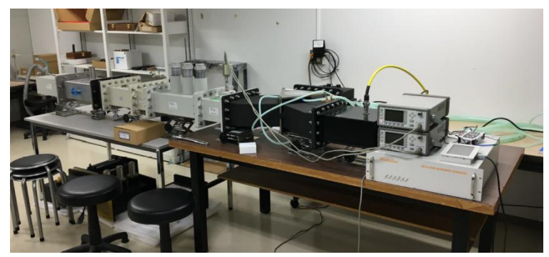
915MHz 1KWシングルモード加熱装置
