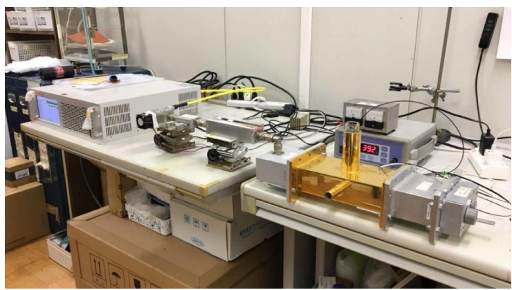
2.45GHz 300Wシングルモード加熱装置
